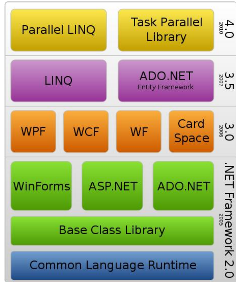
Slika 3. .NET Framework stog
